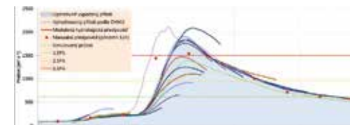
Hydrologické předpovědi průtoku do Orlíka za povodní v červnu 2013.
